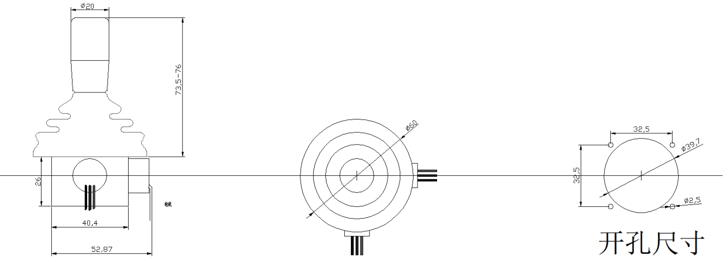
CHD-10LG 外型尺寸图（mm） Appearance size
