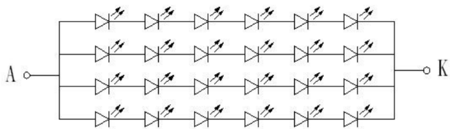
LED 電路圖
